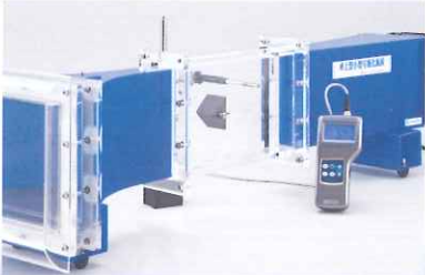
風洞実験
